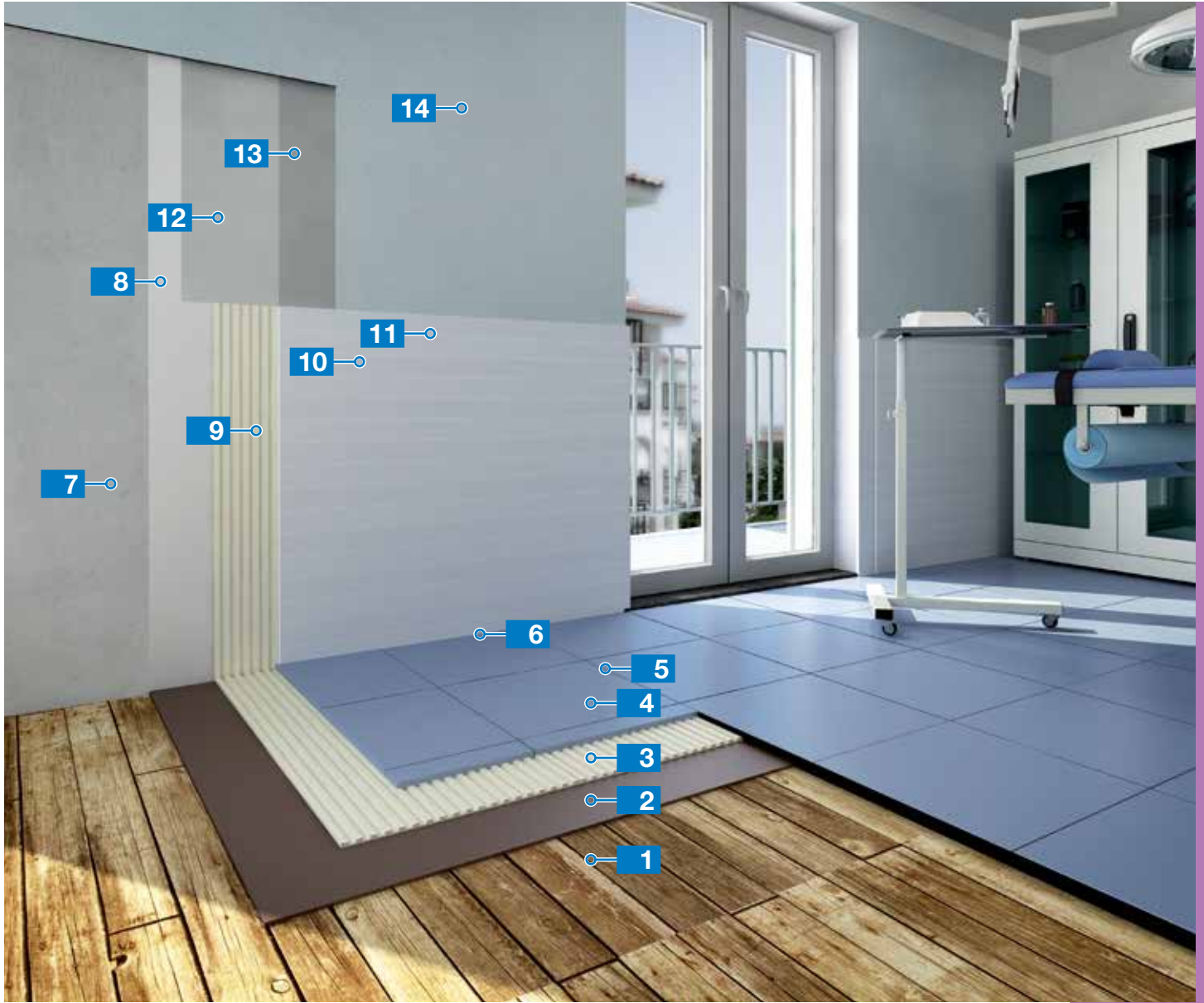
Система для укладки керамической плитки на существующее деревянное покрытие System for the installation of ceramic tiles on existing wooden flooring
