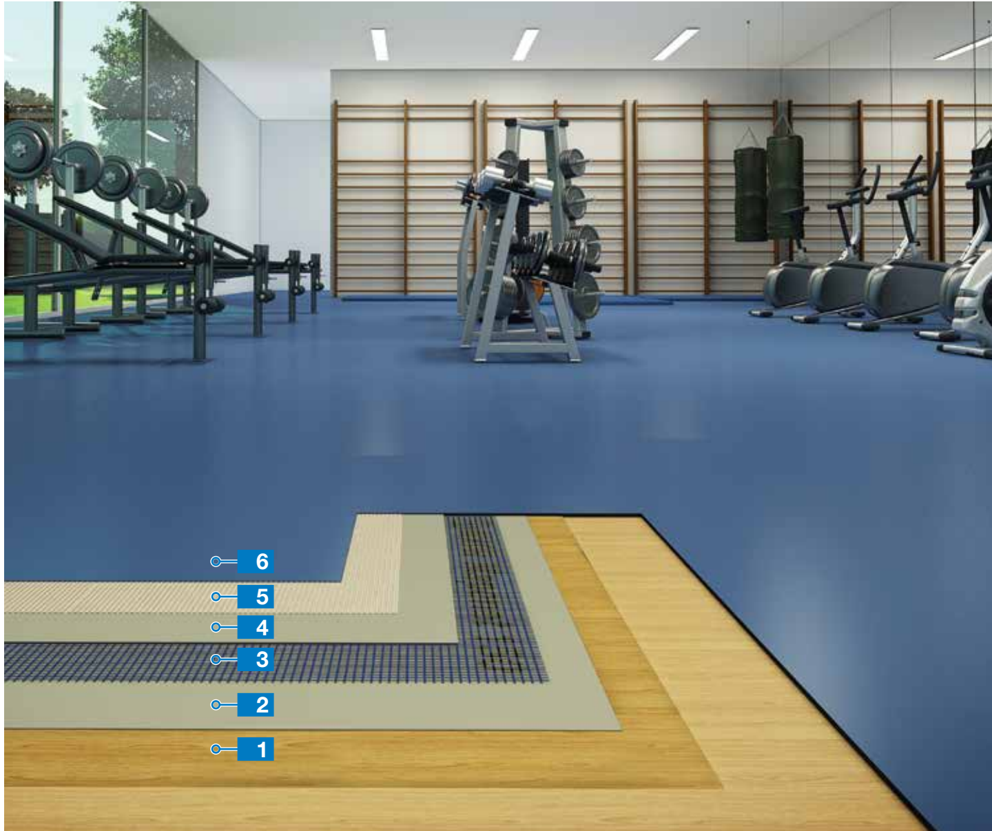
Система для укладки спортивных ПВХ покрытий на основания из многослойной фанеры System for laying PVC sports flooring on plywood substrate
